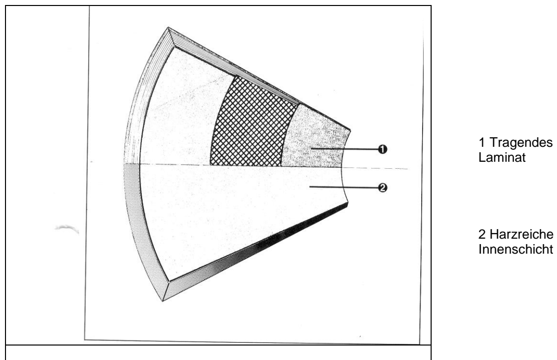
Wandaufbau von Fiberpipe Wickelrohren aus Epoxid- oder Vinylesterharz.
